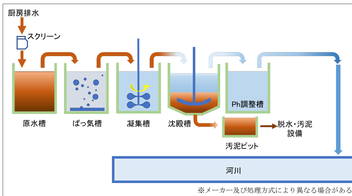
図. 代表的な厨房除害施設処理フロー図
