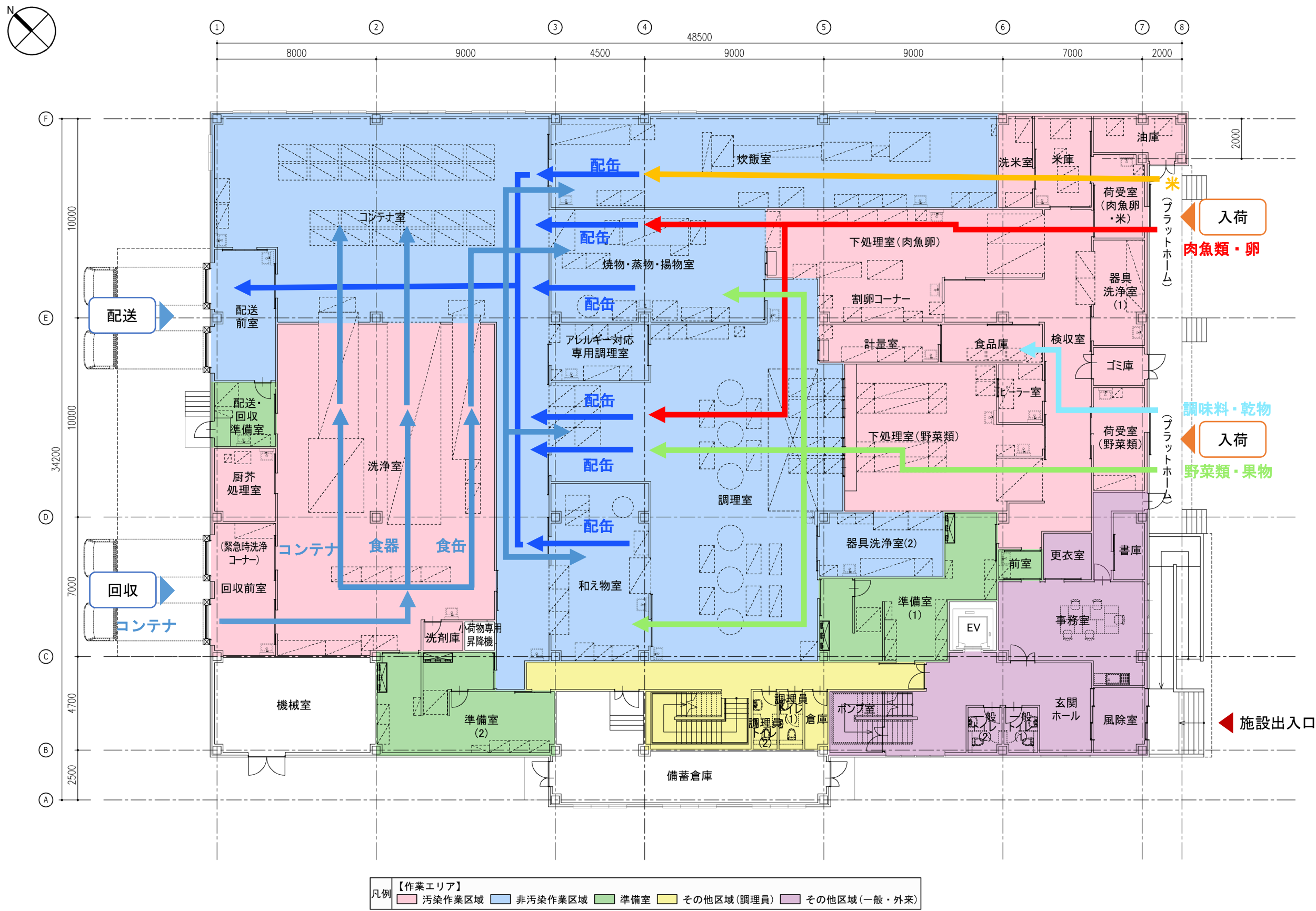
(1) 1階平面図
