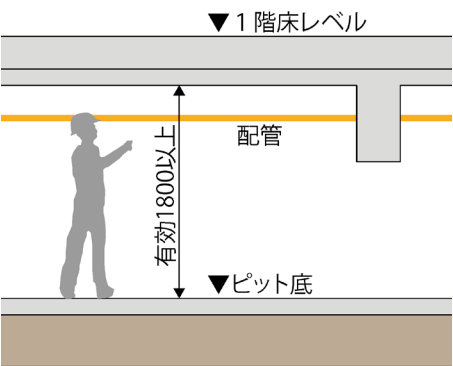
図. 配管ピットのイメージ
