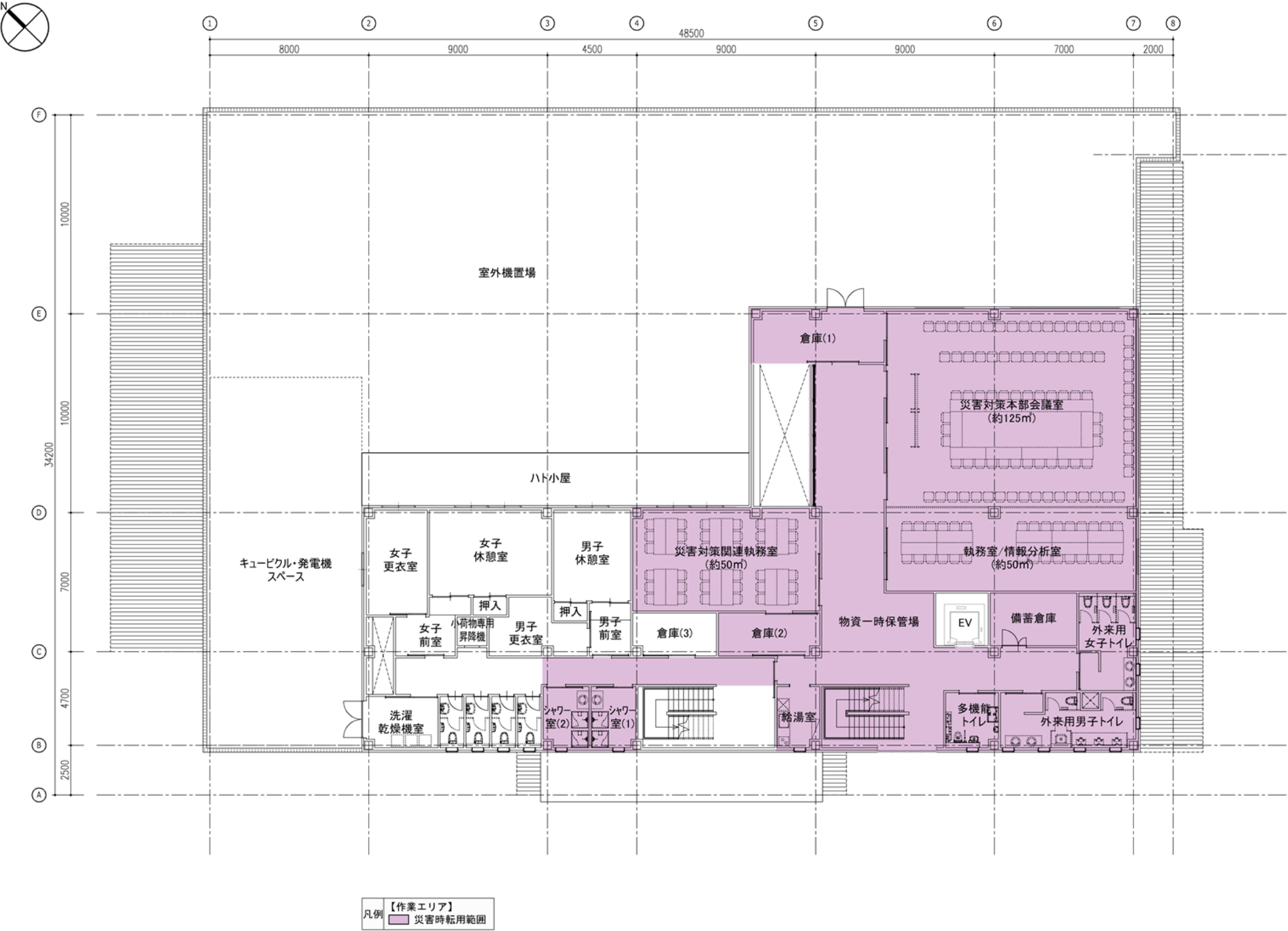
(3) 2階平面図／災害時
