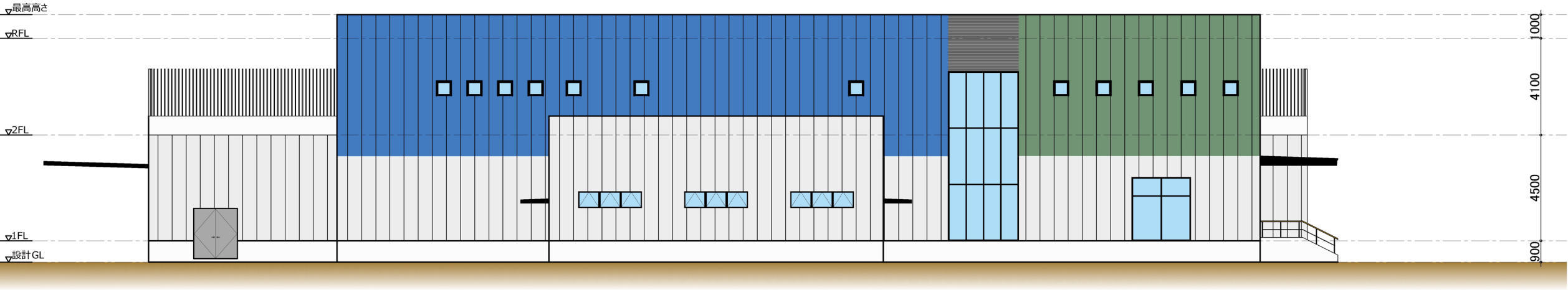
西側立面図
