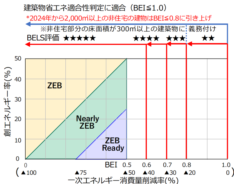
図. ZEB と BELS、省エネ適合性判定の関係
