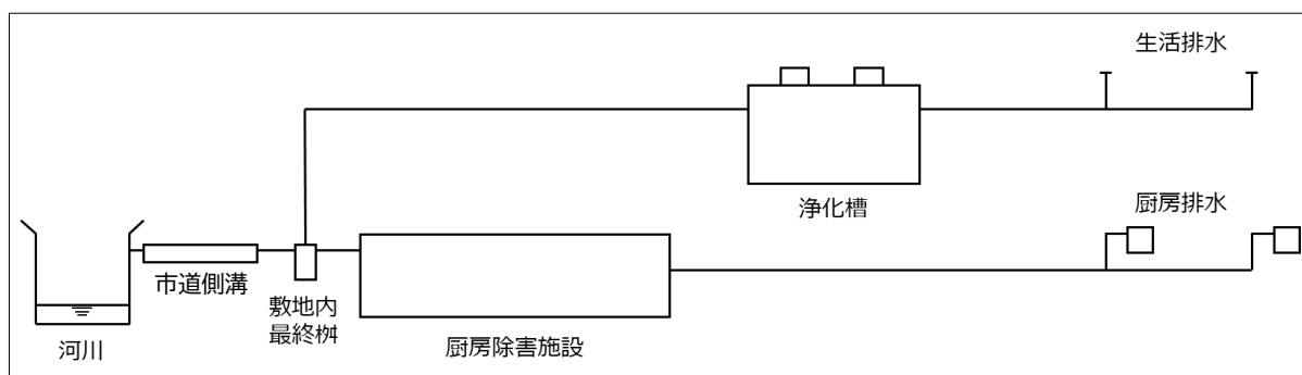
図. 排水処理フローイメージ
