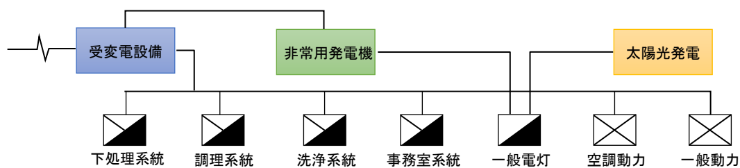
図. 災害時の機能維持を可能とする多重電源
