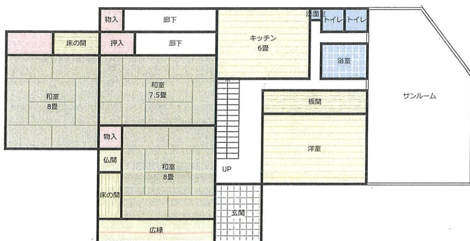
2 階 縮尺 1/150
